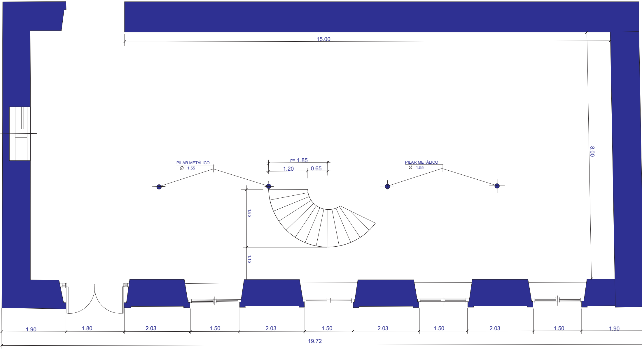
PLANTA BAJA
